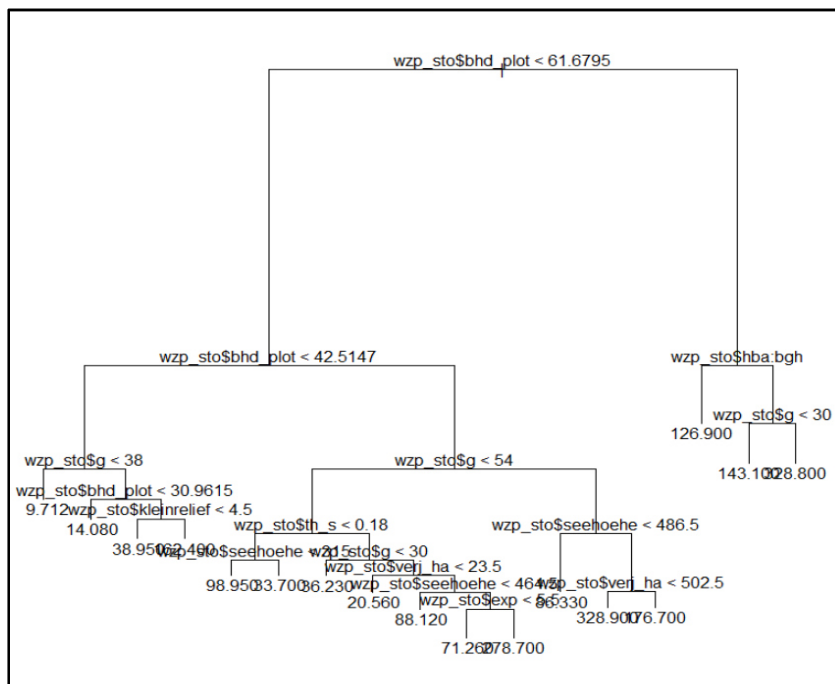
Abb. 22: Aufbau eines beispielhaften Regressionsbaums für die Einflussfaktoren auf den CCF.
